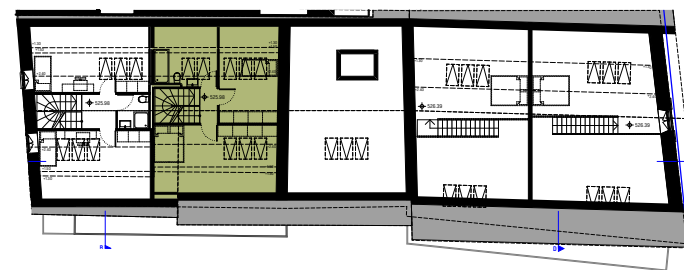
3 ème étage
